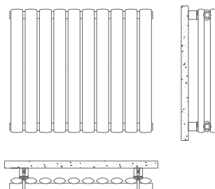
Ellipsis 1 - Design der Rohrenden
