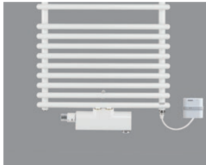
Perfekte Anschlusstechnik für Fußbodentemperierung und Badwärmer mit MF-Ventil. Sommerbetrieb mit Elektroheizstab ZEPELA.
