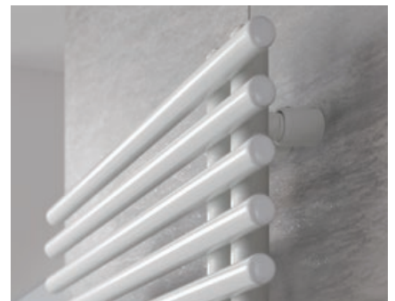
Asymo Metallische Befestigungen an den Sammelrohren erfüllen Anforderungsklasse 3 nach VDI 6036. Im Farbton des Heizkörpers.
